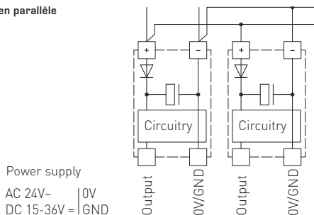
Schéma de raccordement en parallèle
