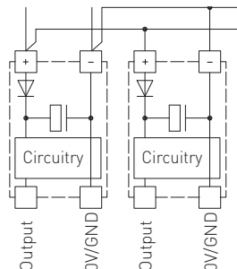
Схема соединения Параллельное подключение
